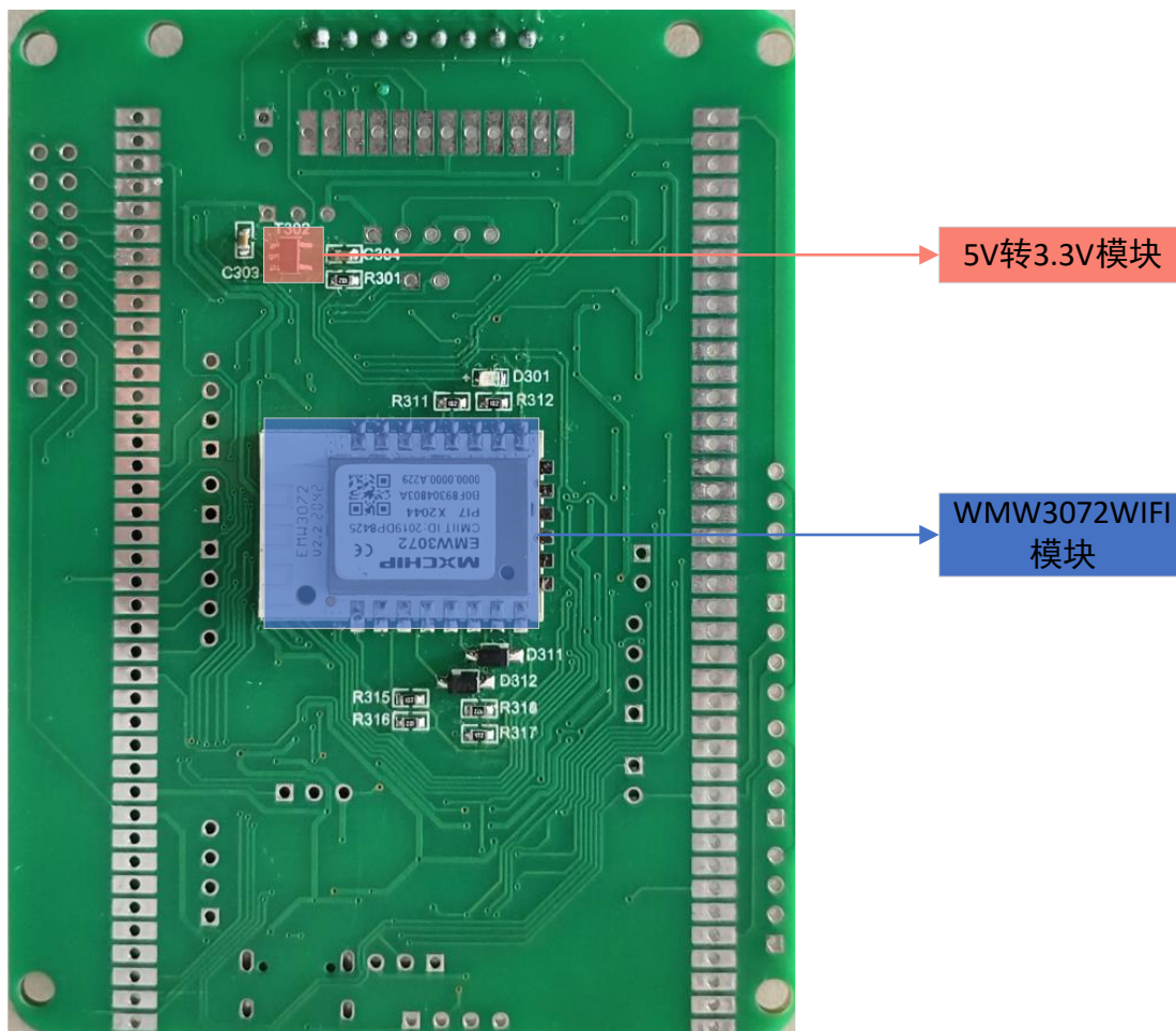
图 2 产品实拍图（背面）
