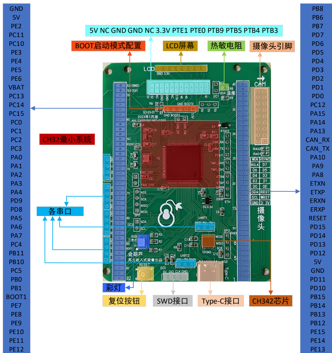
图 1 产品实拍图（正面）
